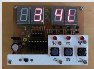
プロトタイプI (バラック)
